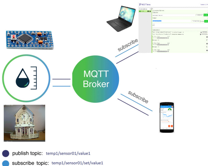
Рис. 4. Диаграмма передачи сообщений
